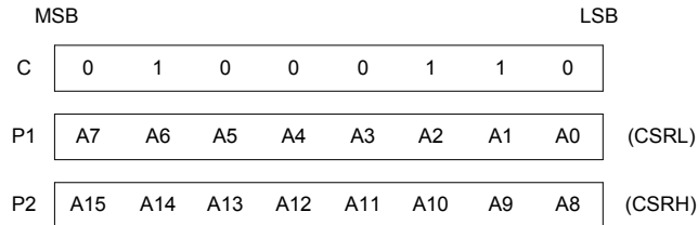
Figure 6-22: CSRW Parameters
