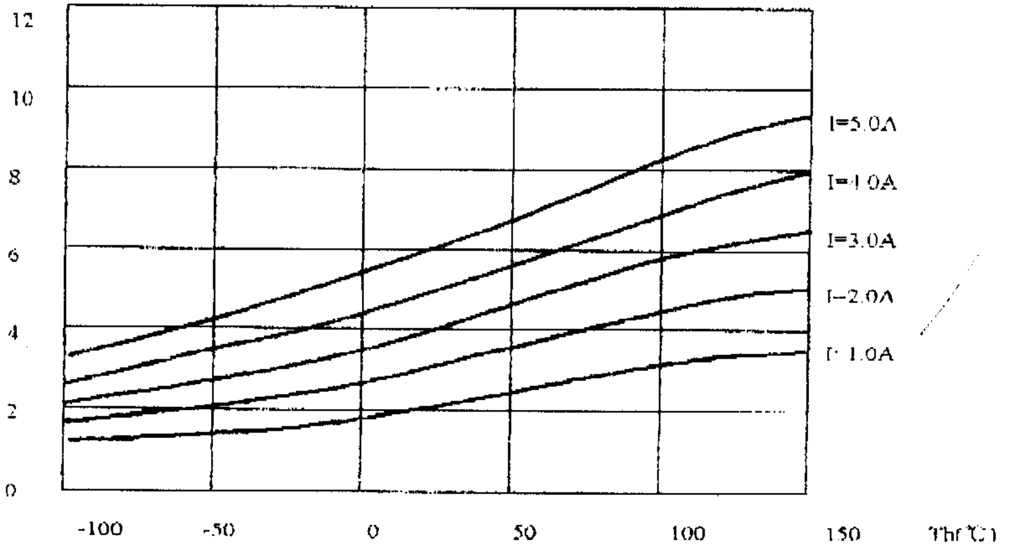
TEC1-7105 Vin - Th 曲线 ΔT = 30°C
