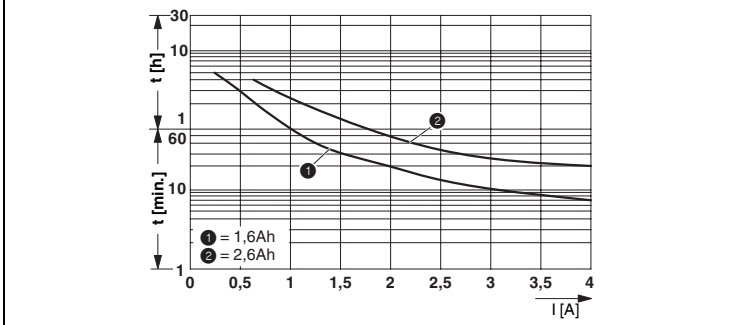
① MINI-BAT 12DC/1,6Ah (Artikel-Nr./Order No./Référence/Código 2866572) ② MINI-BAT 12DC/2,6Ah (Artikel-Nr./Order No./Référence/Código 2866569) Abb./Fig. 5
