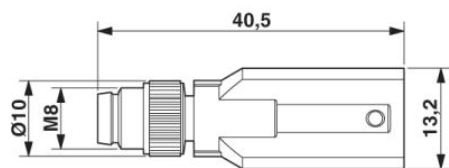
Connettore M8 x 1, distributore a Y
