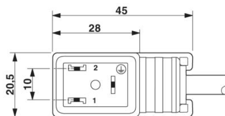
konektor ventilu, konstrukce B
