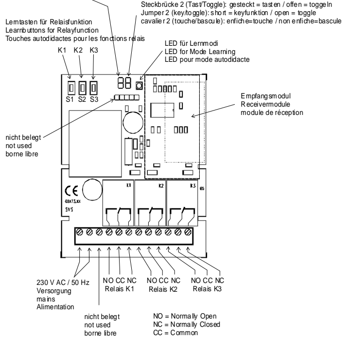
Bild 1: Funktionsübersicht SHR-X L3 Fig. 1: Circuit Board SHR-X L3 Image 1: descriptions des fonctions SHR-X L3
